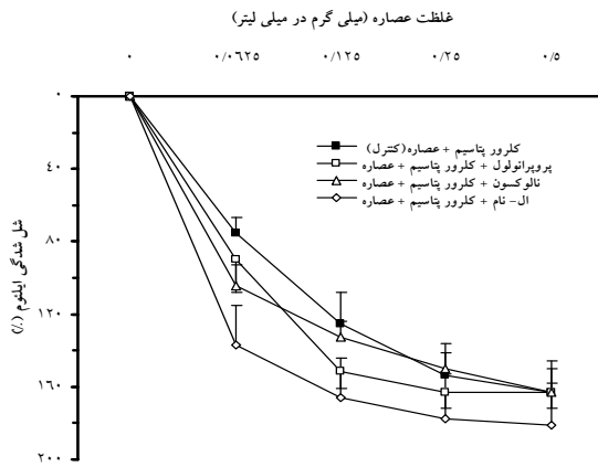
نمودار شماره ۲: مقایسه عملکرد مهاری عصاره آبی الکلی برگ شیرین بیان بر انقباض ناشی از کلرور پتاسیم (۶۰mM) قبل و بعد از اینکوبه کردن ایلئوم با پروپرانولول (۱μM)، نالوکسون (۱μM) و (L-NAME ۱۰۰μM).
