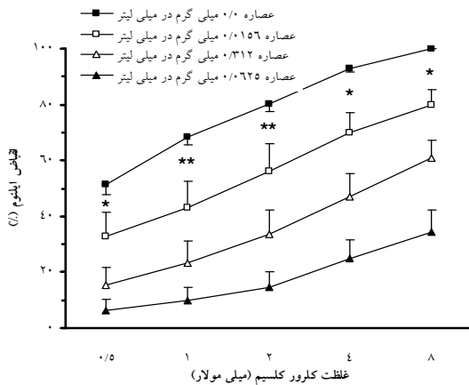
نمودار شماره ۳: مقایسه عملکرد انقباضی غلظتهای مختلف کلرور کلسیم (در محلول تایرود بدون کلسیم دارای غلظت زیاد کلرور پتاسیم) در غیاب و پس از ۳ دقیقه حضور غلظت های مختلف عصاره آبی الکلی برگ شیرین بیان بر ایلئوم موش صحرائی.
