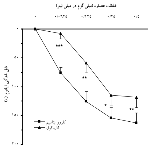
نمودار شماره ۴: مقایسه اثر ضد انقباضی غلظت های تجمعی عصاره آبی الکلی برگ شیرین بیان بر انقباض ناشی از کلرور پتاسیم (۶۰mM) و کارباکول (۱۰μM) در ایلئوم موش صحرائی. * P < 0.05 ، ** P < 0.01 و *** P < 0.001 . اثر ضد انقباضی عصاره بر انقباض ناشی از کلرور پتاسیم قوی تر می باشد (ANOVA دو طرفه، P < 0.001 ).
