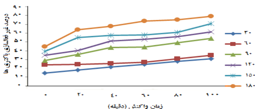
نمودار شماره ۱: روند غیرفعالسازی باکتری ها در مقادیر مختلف محلول نانو نقره بر حسب زمان واکنش
